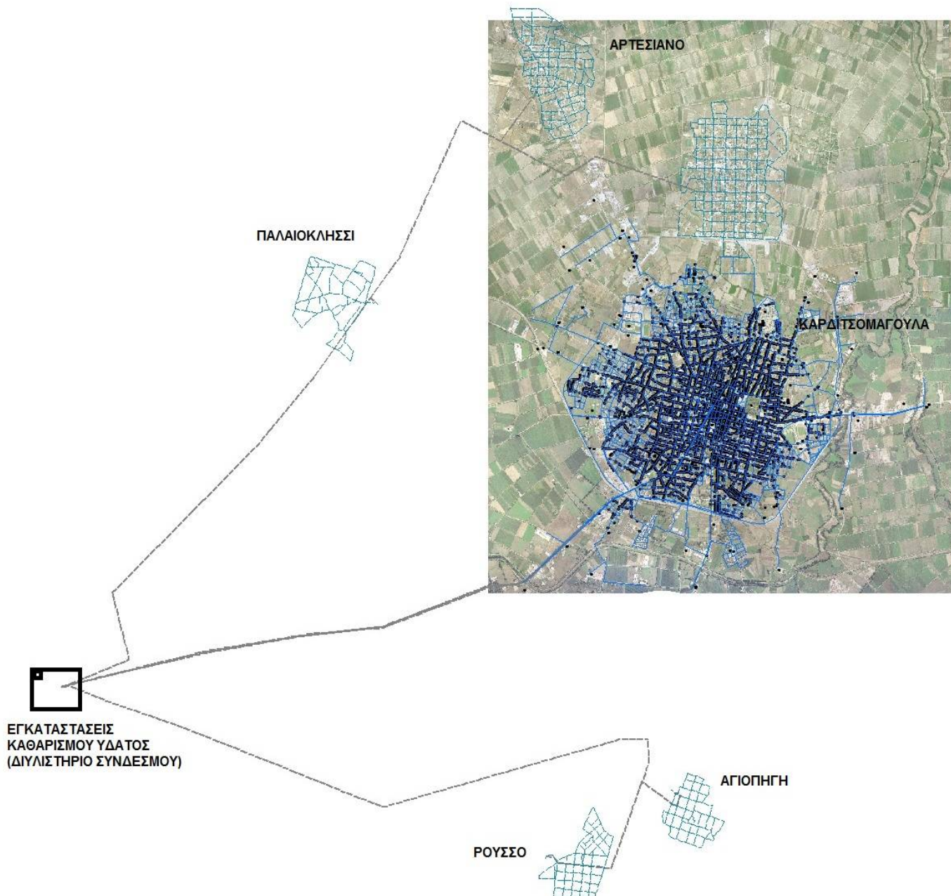
Οριζοντιογραφία δικτύου ύδρευσης Δ.Ε.Καρδίτσας
